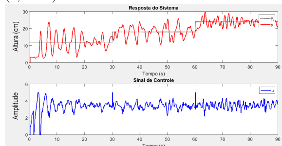
Figura 8: Resposta do sistema a degrau crescente (2, 3 e 4)
