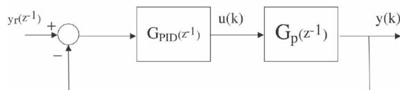
Figura 3: Malha de controle clássica PID
