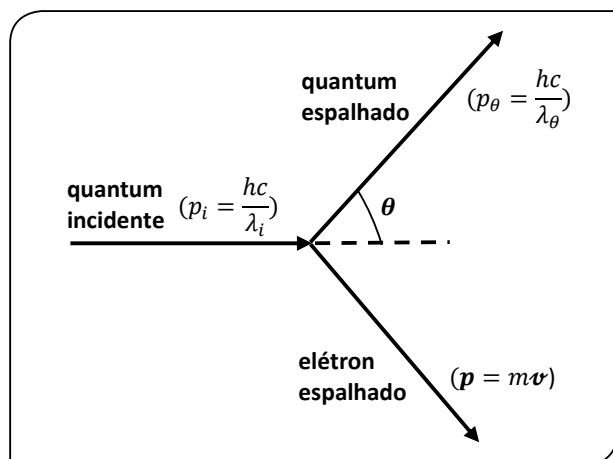
Figura 2. Efeito Compton.
