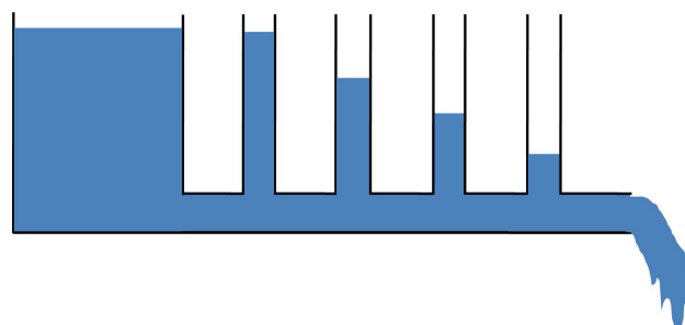
Figura 6. Escoamento de um líquido real.
