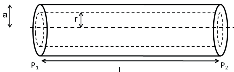
Figura 8. Fluido real que se escoar através de um tubo de comprimento L sob efeito de uma diferença de pressão P_1 - P_2 .
